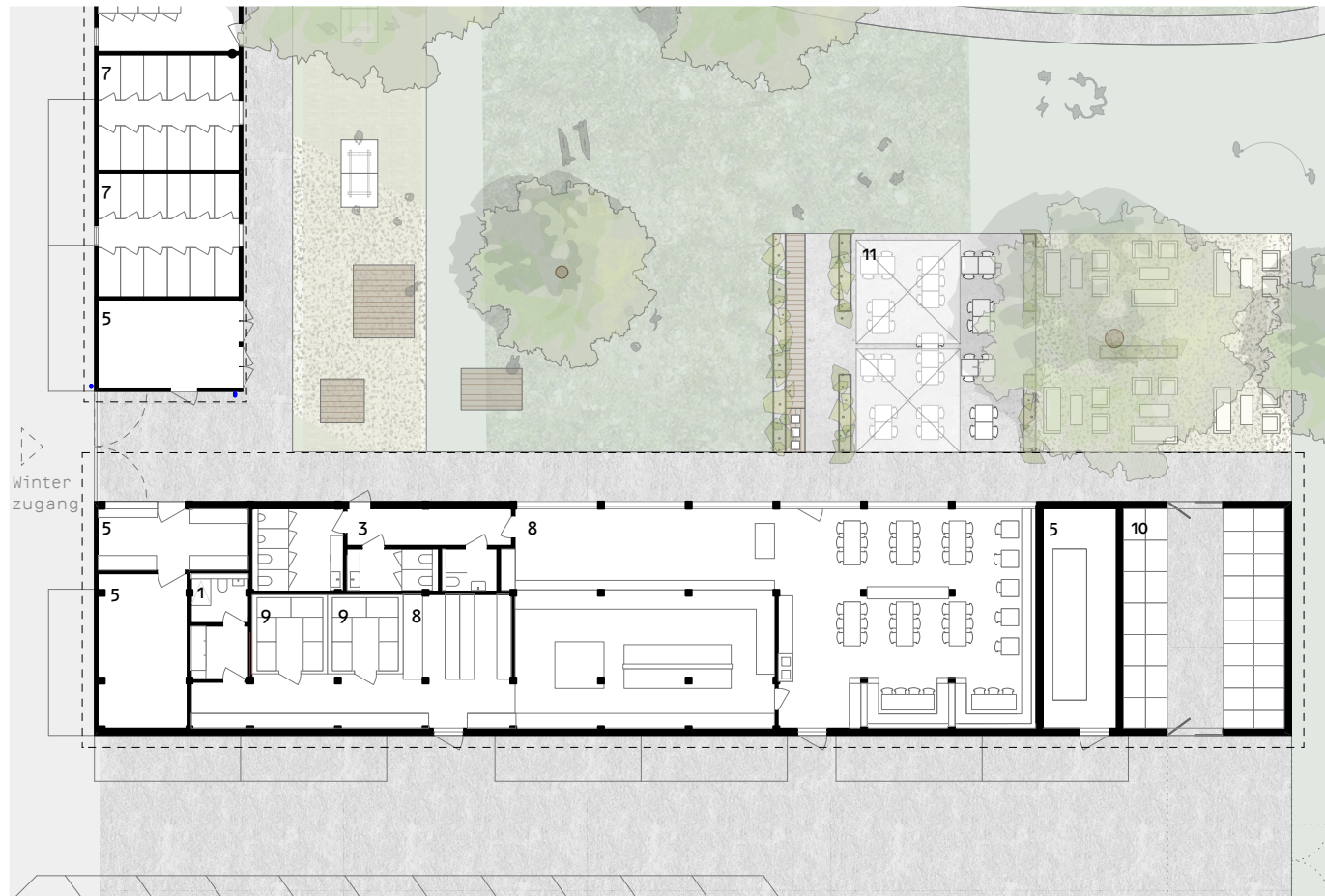
Erdgeschoss Gebäude B+C
