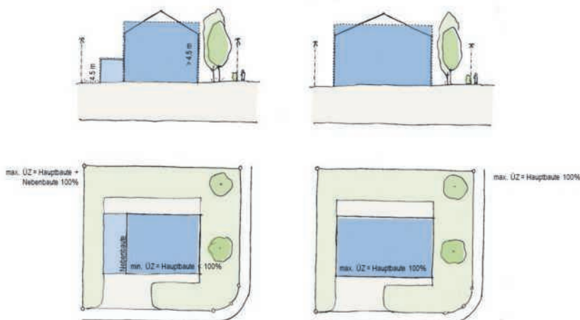
Minimale und maximale Überbauungsziffer (ÜZ) für Haupt- und Nebenbauten
