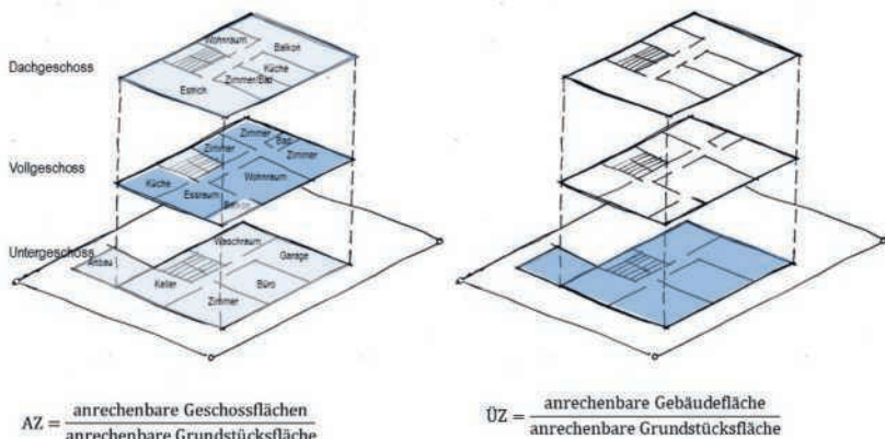
Unterschied zwischen Ausnutzungsziffer (AZ, links) und Überbauungsziffer (ÜZ, rechts)
