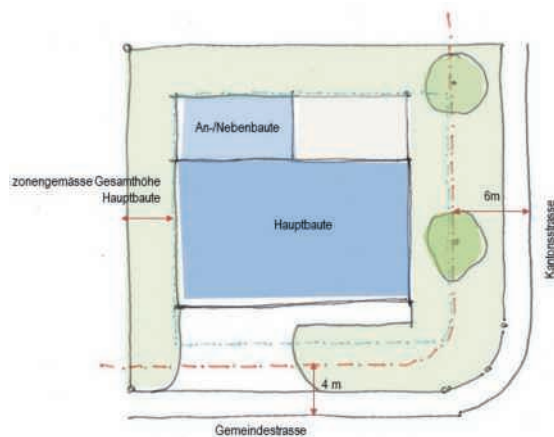
Strassen- und Grenzabstände
