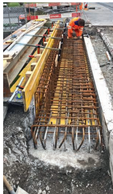
Die Strasse über den Mühlebach wurde um einen Meter verbreitert und im November wurde das erste Kreiselsegment betoniert (unten). Bilder zvg
